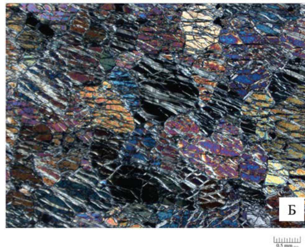
Рис. 2. Фотография шлифа G-19/4. Неизмененные дуниты Инаглинского массива, серпентинизированные по плоскостям расщепления, динамометаморфизованные без новообразований других минералов
