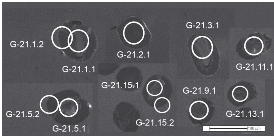
Рис. 7. Катодолюминесцентное изображение цирконов из гнейсов гранат-кварц-кордиеритовых иенгской серии, вмещающих плутон дунитов Инаглинского массива
