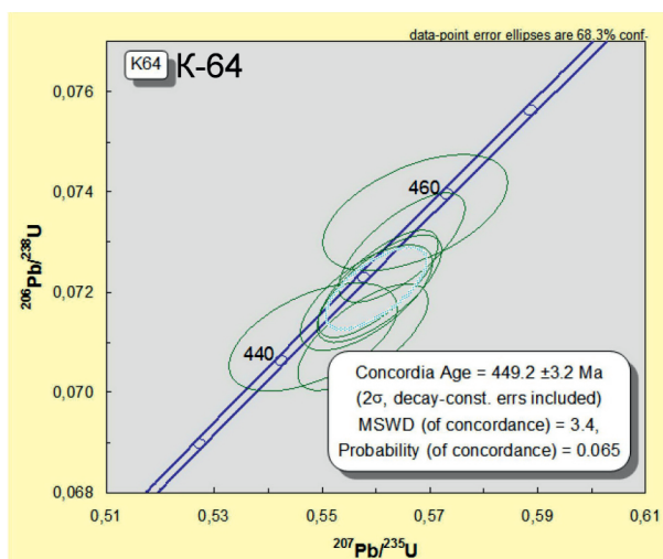
Рис. 3. Диаграммы с конкордиями для цирконов «рудных порфиров» сорского комплекса (Сорский массив, Сорское молибденовое месторождение)
