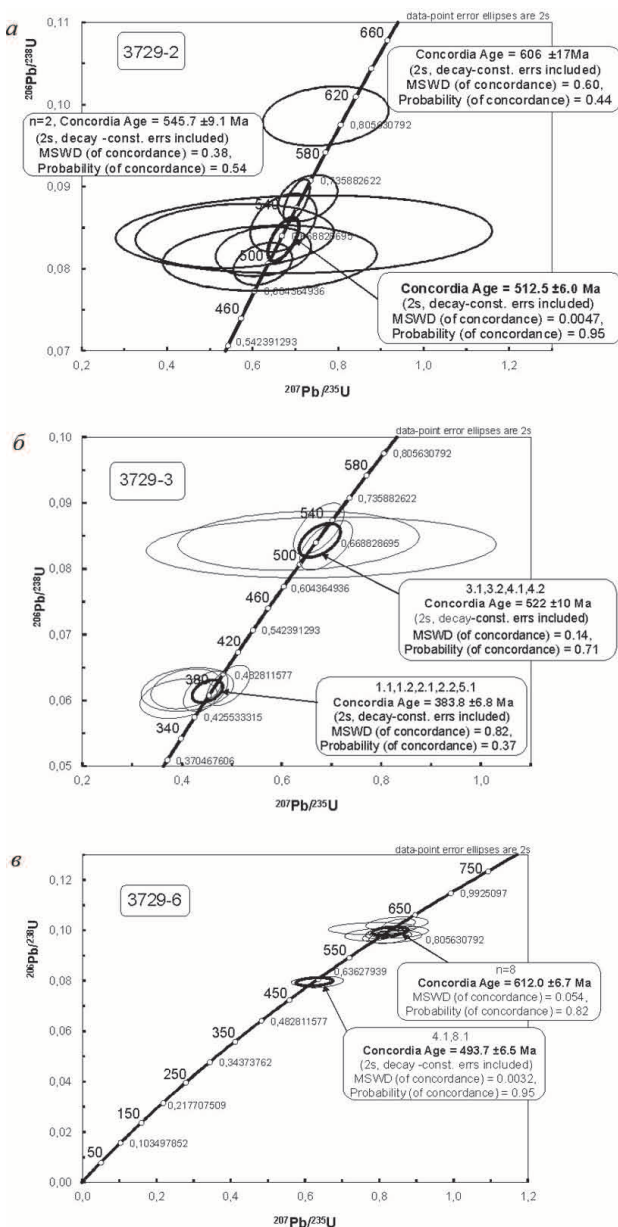
Рис. 10. U-Pb диаграмма с конкордией для цирконов из тектонического микстита на контакте верхнехарьейской и ханмейхойской свит (ручей Ступенчатый)
