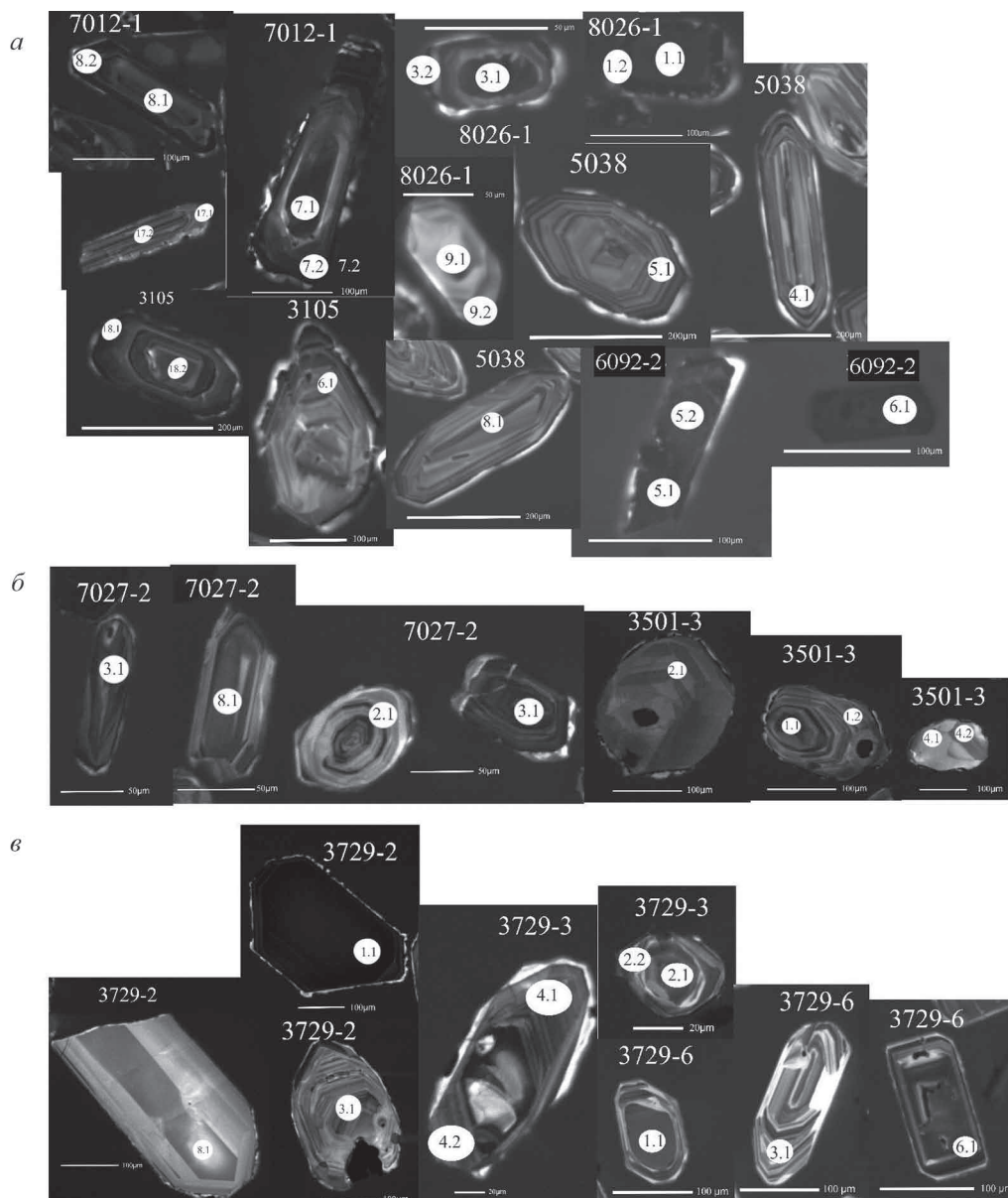
Рис. 4. Изображение цирконов в катодолюминесцентном свете
