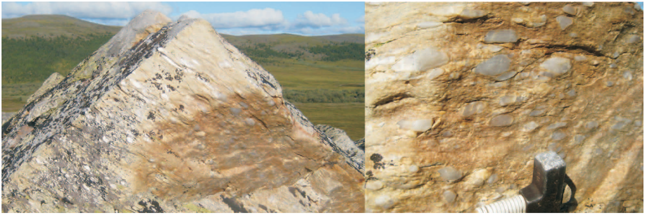
Рис. 3. Псевдогалки кварца в полевошпатово-кварцевых породах (ручей Лаптаяха)
