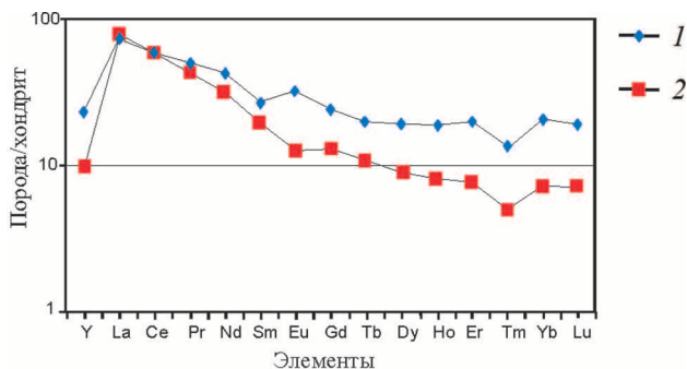
Рис. 9. Спайдер-диаграмма распределения редкоземельных элементов в обломках 1 – эпидотизированных метадiorитов (3729-3) и 2 – матрикса тектонического микстита (3729-2) с контакта ханмейхойской и верхнехарьейской свит (ручей Ступенчатый)
