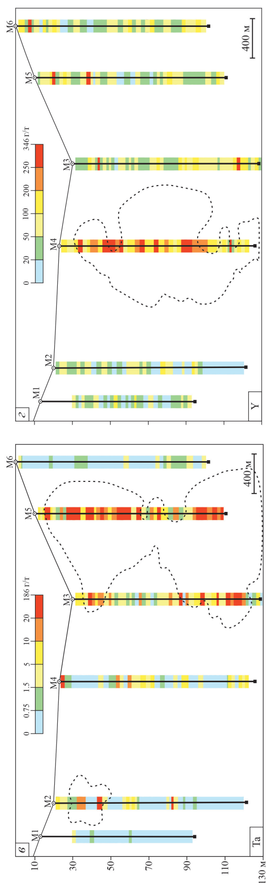
Рис. 6. Схематический геологический разрез Мальджангарского карбонатного массива с контурами распределения элементов: LREE (а), Nb (б), Ta (в) и Y (г). 1 – раннепротерозойские метаморфические породы верхнекамбрийского комплекса; 2 – кальцитовые карбонаты; 3 – доломитовые карбонаты; 4 – кальцит-доломитовые карбонаты; 5 – четвертичные и неоген-четвертичные отложения; 6 – потенциальные разрывные нарушения. Пунктирной линией показаны геохимические аномалии
