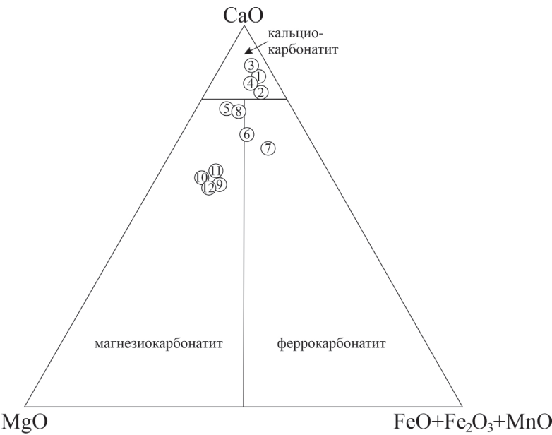
Рис. 3. Классификация и номенклатура карбонатитов [38]
