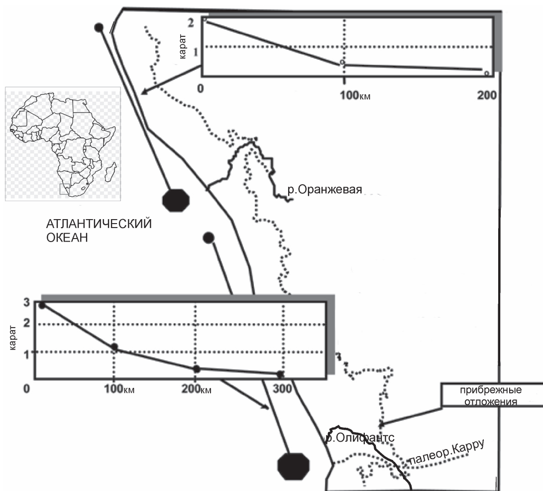
Рис. 1. Распределение среднего размера алмазов в прибрежных алмазоносных отложениях Атлантического океана [3]
