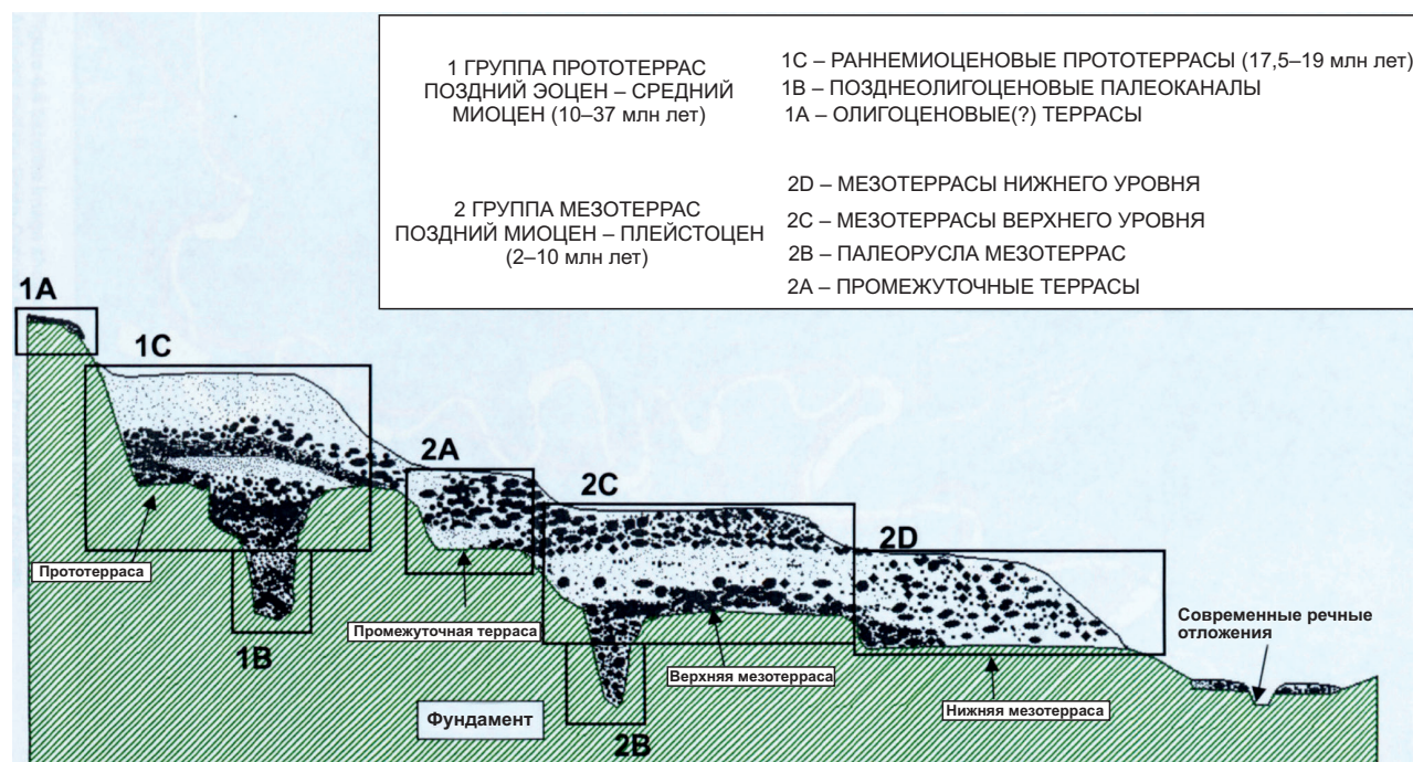
Рис. 3. Прото- и мезотеррасы нижнего течения р. Оранжевая [11]
