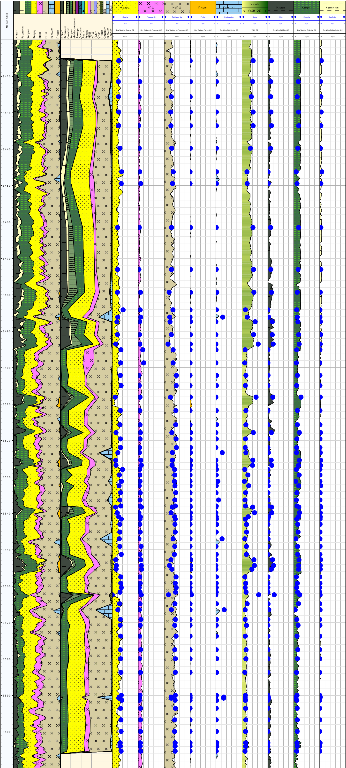
Рис. 4. Сопоставление минерального состава по результатам обработки данных АИНК-ПЛ и рентгеноструктурного анализа по скв. 1 Fig. 4. Comparison of mineral composition after the AINK-PL results interpretation and X-ray diffraction analysis in well 1
