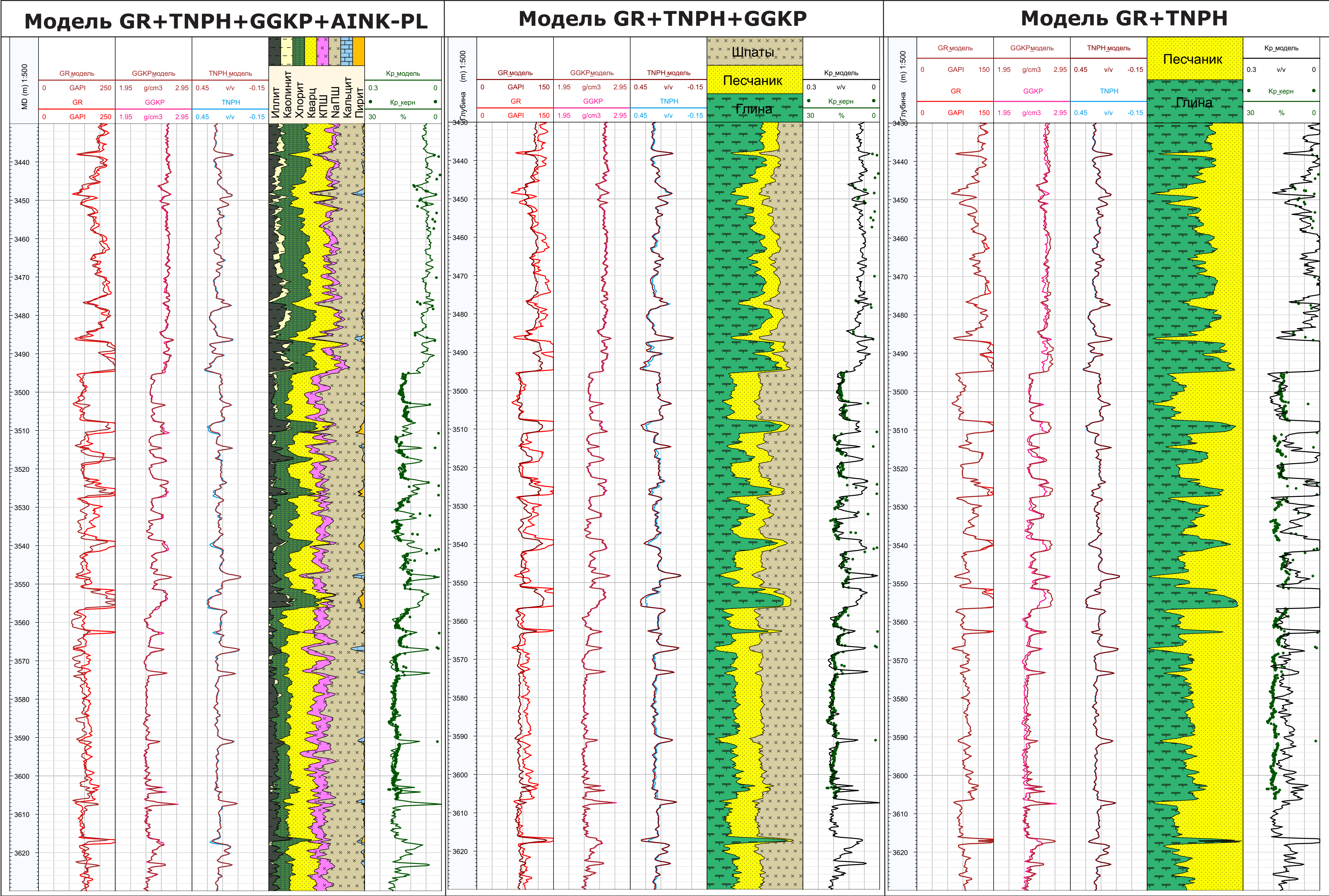
Рис. 7. Сопоставление результатов моделирования по скв. 1 Fig. 7. Comparison of modeling results in well 1
